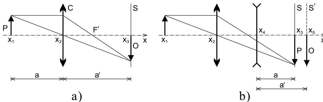
Obrázek 1: Měření ohniskové vzdálenosti a) spojky a b) rozptylky
