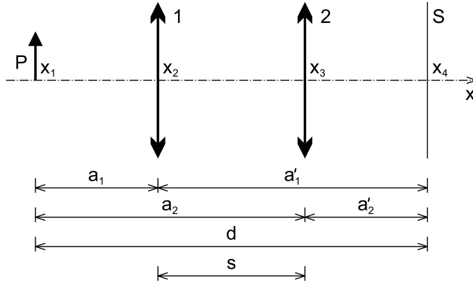
Obrázek 2: Besselova metoda
